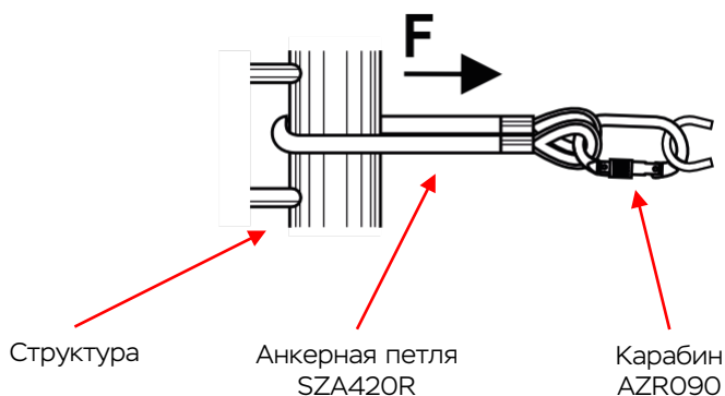
Рис. 3 Вид системы, закрепленной за стационарные анкерные устройства
